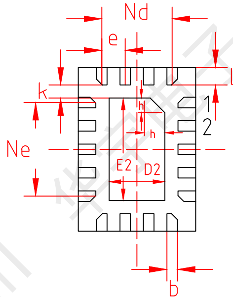
BOTTOM VIEW 背视图
