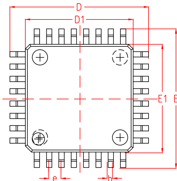
TOP VIEW 正视图
